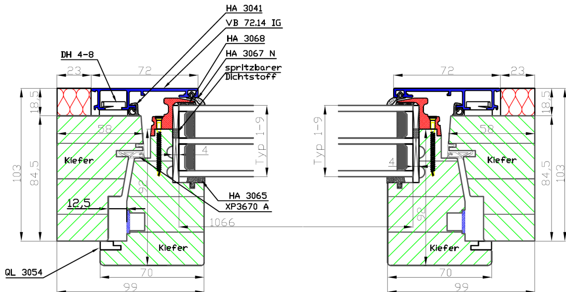
Bild 4 Horizontalschnitt, geprüft wurde mit 8 VSG/18/4/18/6 Verglasung (Typ 4)
